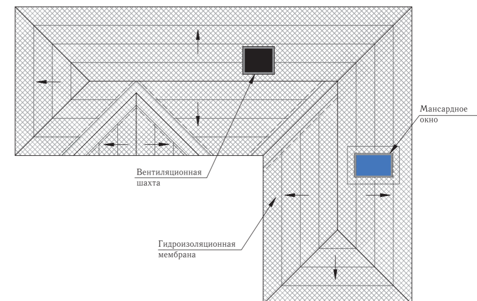
Рис. 4.14. Гидроизоляция по всей поверхности крыши
